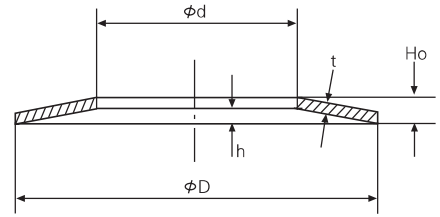
碟形弹簧截面形状
